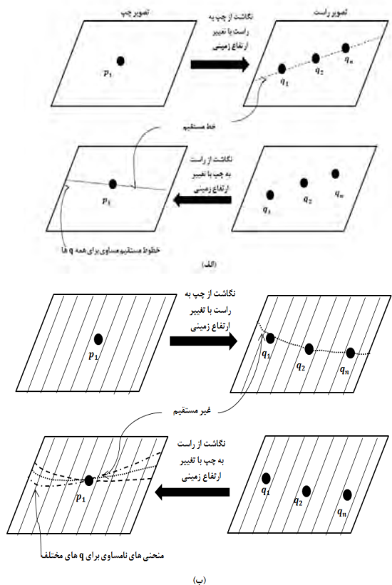
شکل ۳- مقایسه ویژگی های مهم اپی پولاتر در حالت الف) دوربین بر مبنای فریم و ب) دوربین آرایه خطی
