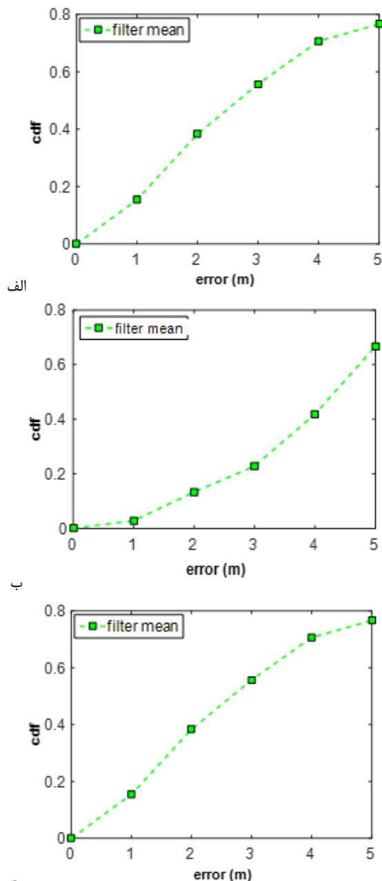
شکل ۱۳- روش شبکه عصبی برای سناریو ۲. الف) ۳۵ ورودی با میانگین‌گیری از نمونه‌ها در هر نقطه ب) ۱۰۵ ورودی و ۳ نمونه در هر نقطه ج) ۳۵۰۰ ورودی و ۱۰۰ نمونه در هر نقطه
