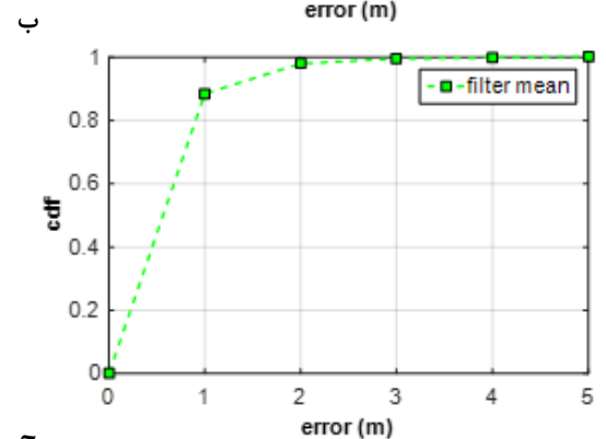
شکل ۱۱- روش شبکه عصبی برای سناریو ۱ الف) ۱۶ ورودی با میانگین‌گیری از نمونه‌ها در هر نقطه ب) ۹۶ ورودی و ۶ نمونه در هر نقطه ج) ۱۶۰۰ ورودی و ۱۰۰ نمونه در هر نقطه
