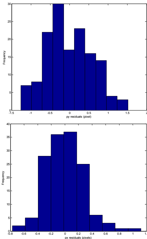
شکل ۱۲- هیستوگرام باقیمانده‌های py (بالا) و px (پایین) پس از اجرای توجیه نسبی یکجا (معادله ۱۵)، بر روی ۱۴۴ نقطه‌ی اندازه‌گیری شده در اپوکهای (۲۰۰۹/۲۰۰۸)
