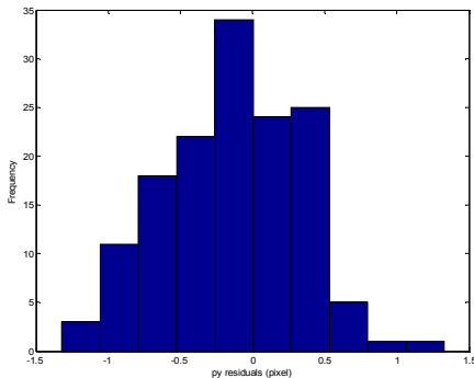
شکل ۲۲- هیستوگرام مقادیر py پس از حل توجیه نسبی با معادله- ی (۱۶) برای نقاط چک با ضرائب بدست آمده بر روی نقاط گروبر
