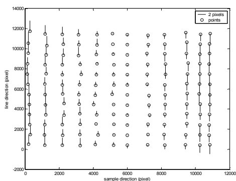
شکل ۹- px باقیمانده پس از حذف اثر BX .
