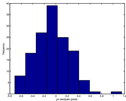
شکل ۲۳- هیستوگرام مقادیر px پس از حل توجیه نسبی با معادله- ی (۱۶) برای نقاط چک با ضرائب بدست آمده بر روی نقاط گروبر
