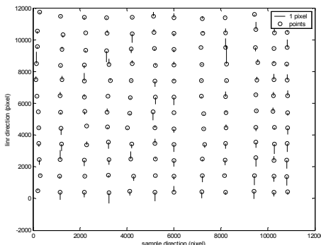
شکل ۲۱- مولفه‌های px پس از حل توجیه نسبی با معادله‌ی (۱۶) برای نقاط چک با ضرائب بدست آمده بر روی نقاط گروبر
