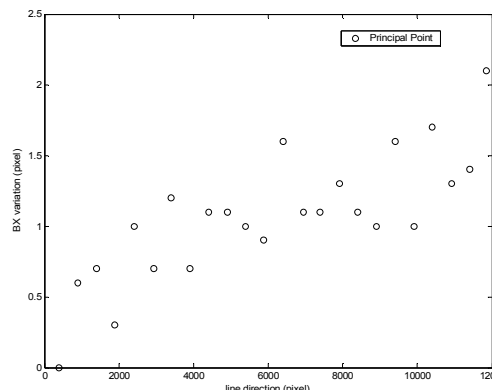
شکل ۷- دریفت BX در جهت حرکت ماهواره برای تصاویر اپوکهای ۲۰۰۸ و ۲۰۰۹
